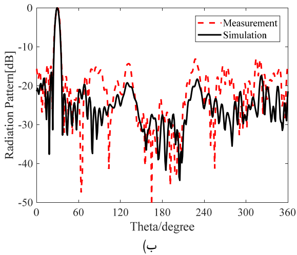
(ادامه) شکل ۱۰- مقایسه نتایج شبیه سازی و ساخت پرتو میدان دور نرمالیزه (الف) در جهت (\theta=0^\circ, \phi=90^\circ) با قطبش عمودی (ب) در جهت (\theta=90^\circ, \phi=90^\circ) و (\theta=30^\circ, \phi=0^\circ) با قطبش افقی.
