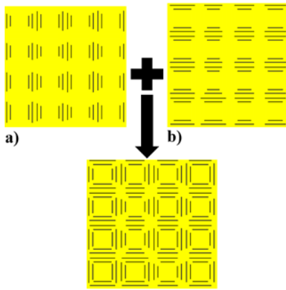
شکل ۶- (a) طراحی مؤلفه‌ی عمودی برای پرتو در جهت \theta = 0^\circ و \phi = 90^\circ طراحی مؤلفه‌ی افقی برای پرتو در جهت \theta = 90^\circ و \phi = 0^\circ ساختار کامل متشکل از عناصر مؤثر در قطبش عمودی و قطبش افقی
