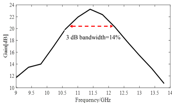
شکل ۷- پهنای باند آنتن آرایه‌ی بازتابی ارائه شده
