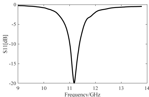
شکل ۵- منحنی مربوط به |S_{11}| تغذیه آنتن آرایه‌ای بازتابنده در حالتی که روبه‌روی بازتابنده قرار دارد
