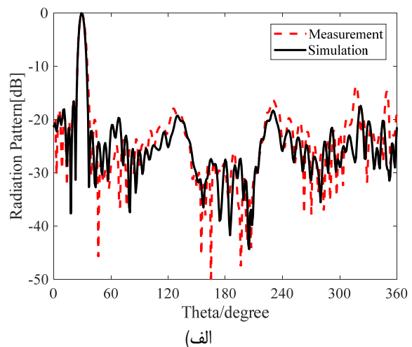
شکل ۱۰- مقایسه نتایج شبیه سازی و ساخت پرتو میدان دور نرمالیزه (الف) در جهت (\theta=0^\circ, \phi=90^\circ) با قطبش عمودی (ب) در جهت (\theta=90^\circ, \phi=90^\circ) و (\theta=30^\circ, \phi=0^\circ) با قطبش افقی.
