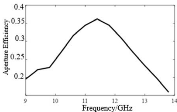
شکل ۸- نمودار بازدهی برحسب فرکانس (فرکانس طراحی ۱۱/۴ GHz)
