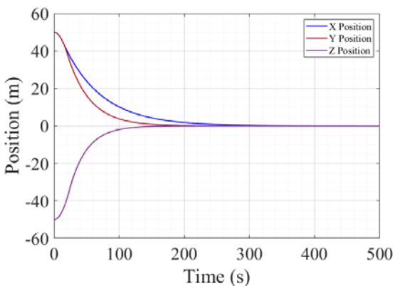
شکل ۱۳- موقعیت فضایی تعقیب کننده (تراست ۵۶ نیوتن)
