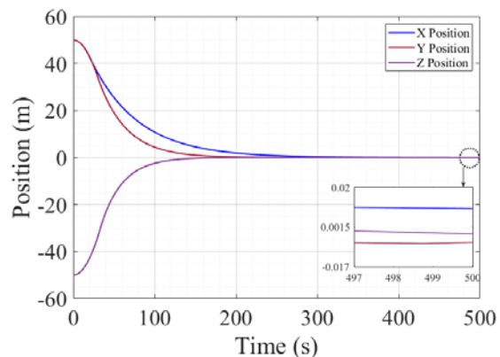
شکل ۵- موقعیت فضایی تعقیب‌کننده
