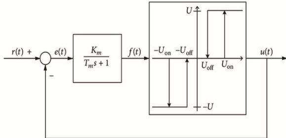
شکل ۲- گسسته‌ساز PWWF
