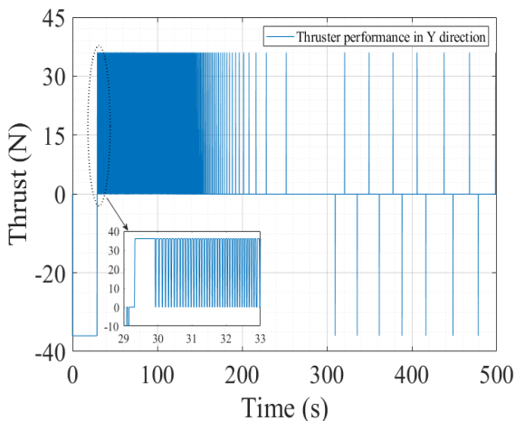
شکل ۷- عملکرد رانشگر در راستای Y
