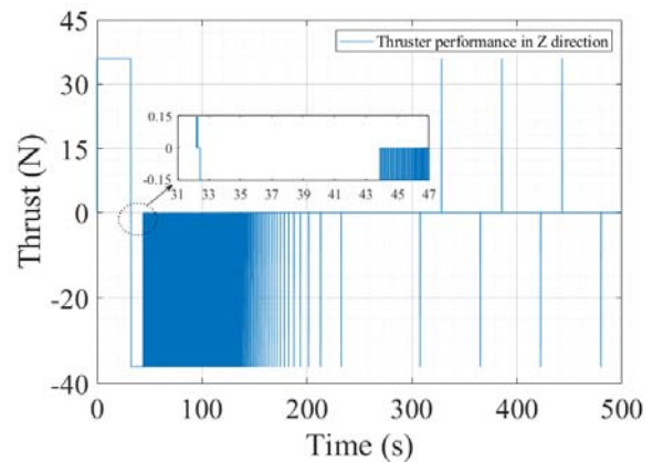
شکل ۸- عملکرد رانشگر در راستای Z
