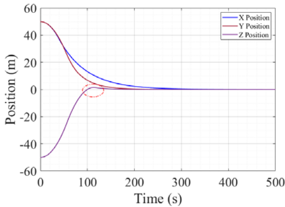
شکل ۱۲- موقعیت فضایی تعقیب کننده (تراست ۱۶ نیوتن)
