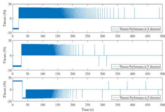
شکل ۱۰- عملکرد رانشگرها در حضور اعمال عدم قطعیت
