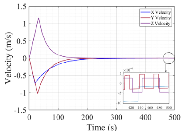
شکل ۹- سرعت فضاییما تعقیب کننده
