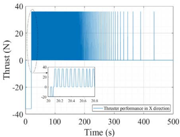
شکل ۶- عملکرد رانشگر در راستای X
