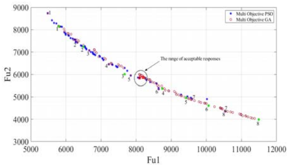
شکل ۴- جبهه پرتو
