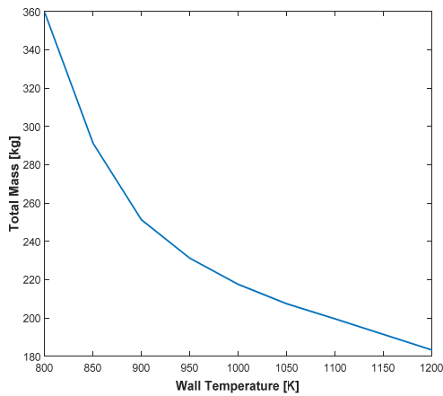
شکل ۵- تغییرات جرم کل با قید دمایی دیواره محفظه احتراق
