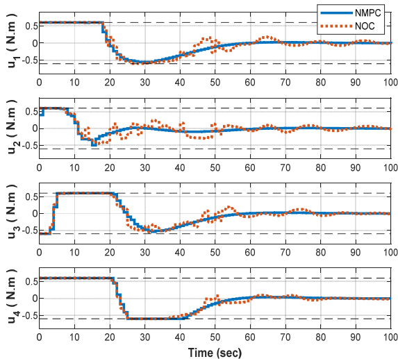
شکل ۲- گشتاور کنترلی با چهار چرخ فعال
