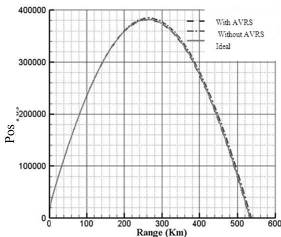
شکل ۱۱- نمودار مقایسه برد جسم پرنده در دو حالت با و بدون AVRS برای اغتشاش ضریب افت المان مسیر سوخت محفظه
