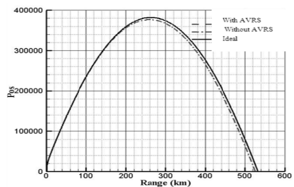
شکل ۱۲- نمودار مقایسه برد جسم پرنده در دو حالت با و بدون AVRS برای اغتشاش دمای پیشران
