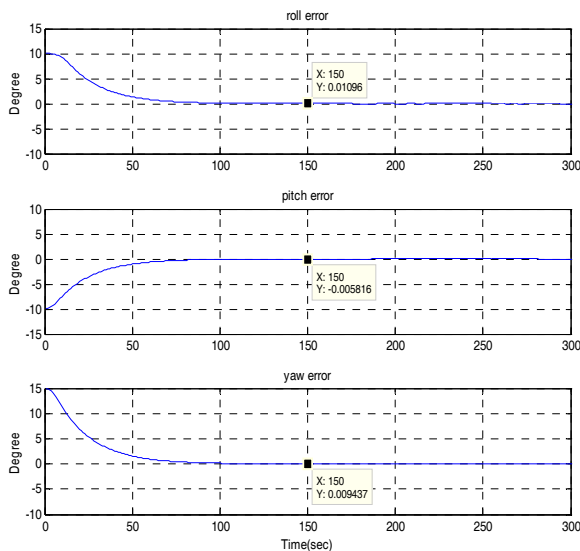
شکل ۷- خطای ردیابی وضعیت حول سه محور رول، پیچ و یابو در صورت بروز عیب چرخ‌های عکس‌العملی ماهواره و عدم جبران‌سازی عیب
