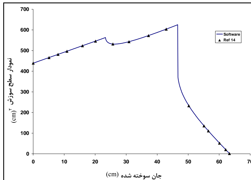
شکل ۱۴- تغییرات سطح سوختن نسبت به جان سوخته شده برای گرین چرخ واگن پنج پر
