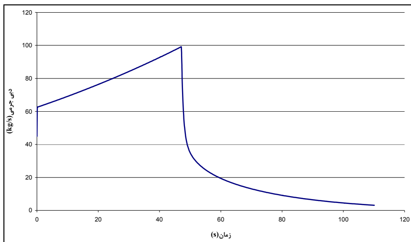
شکل ۱۲- نمودار تغییرات دبی جرمی خروجی از نازل (گرین چرخ واگن)
