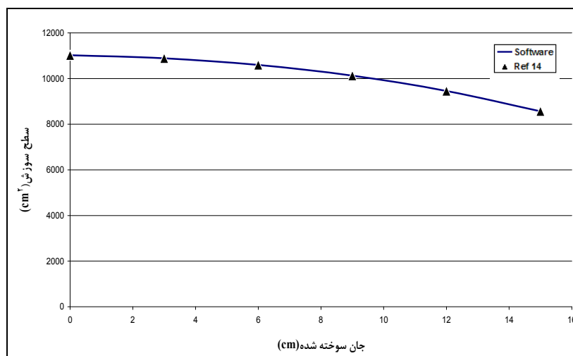
شکل ۱۵- تغییرات سطح سوختن نسبت به جان سوخته شده برای گرین شیاردار سه شیار
