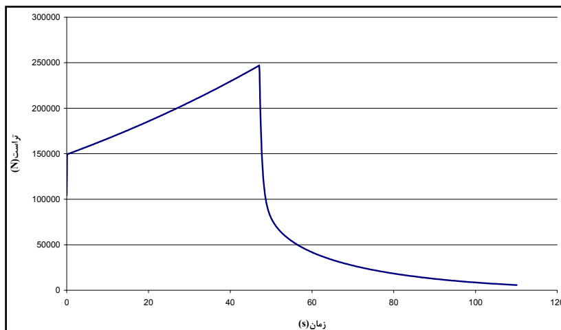
شکل ۱۱- نمودار تغییرات پیشران نسبت به زمان (گرین چرخ واگن)
