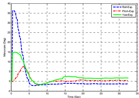
شکل ۷- نمودار زوایای اوپلر در راستاهای رول، پیچ و یاو در آزمایش ۲
