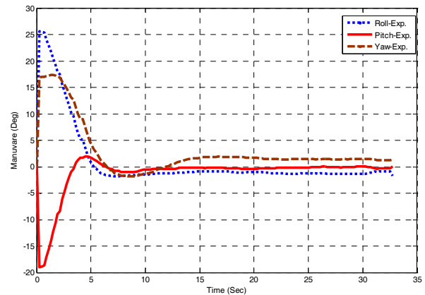
شکل ۳- نمودار زوایای اوایلر در راستاهای رول، پیچ و یاو در آزمایش ۱
