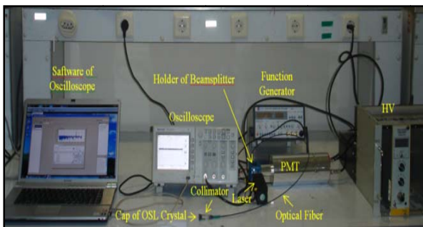
شکل ۸- نمایی از سیستم دزیمتری آزمایشگاهی OSL ساخته شده در دانشگاه صنعتی مالک اشتر اصفهان
