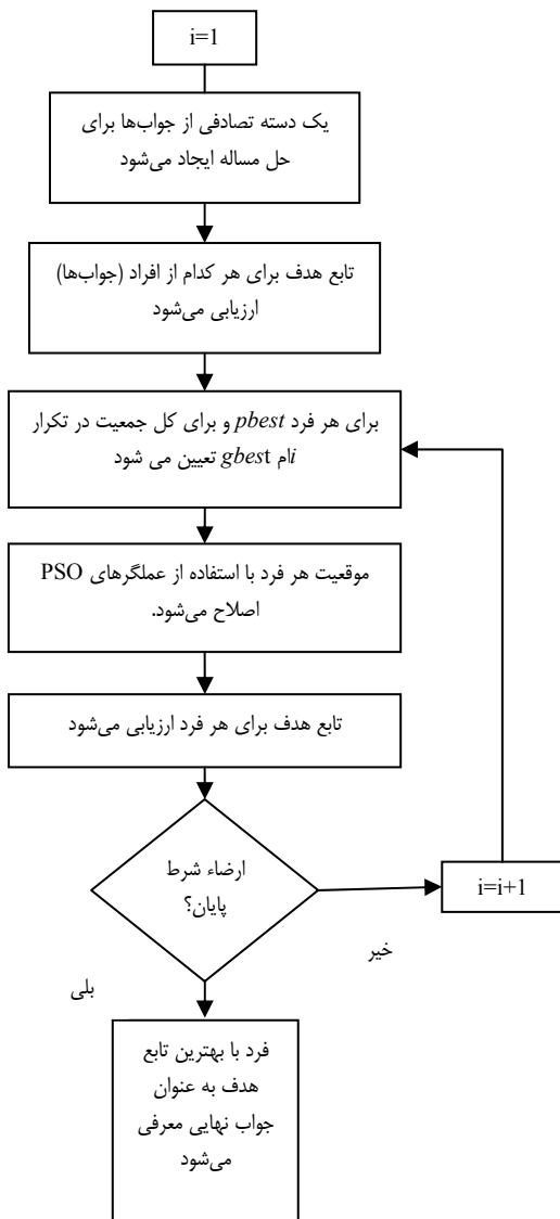
شکل ۳- الگوریتم PSO [۱۰]
