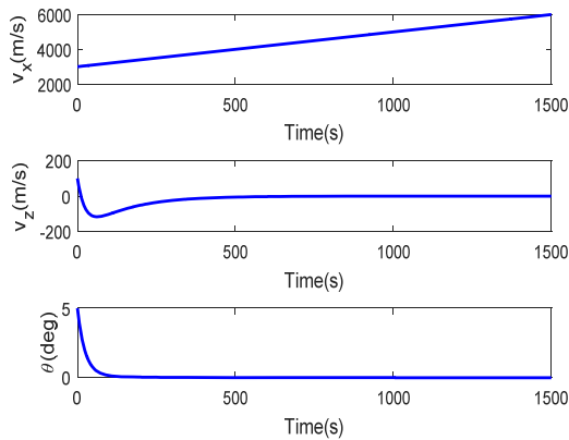
شکل ۲۴- پاسخ زمانی بردارهای وضعیت فضاییما در مرجع [۱۶]
