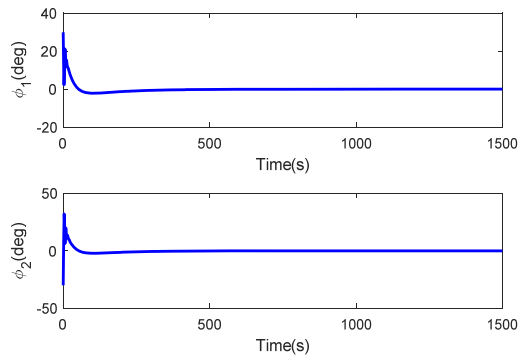
شکل ۱۷- پاسخ زمانی بردارهای وضعیت فضاپیما برای کنترلر لیاپانوف
