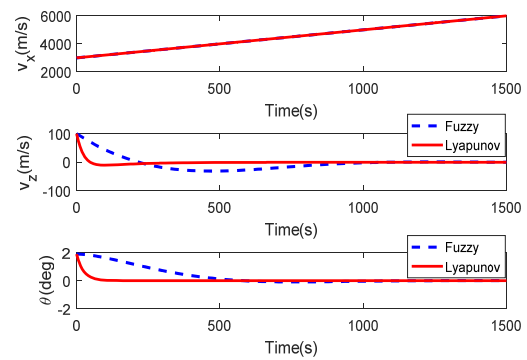
شکل ۲۱- مقایسه پاسخ زمانی وضعیت فضاییما برای کنترلرهای غیرخطی
