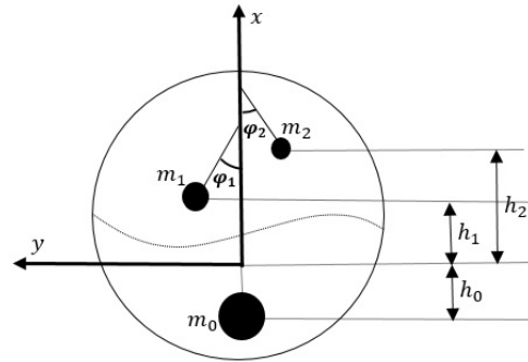
شکل ۲- مدل دو پاندولی تالطم سوخت
