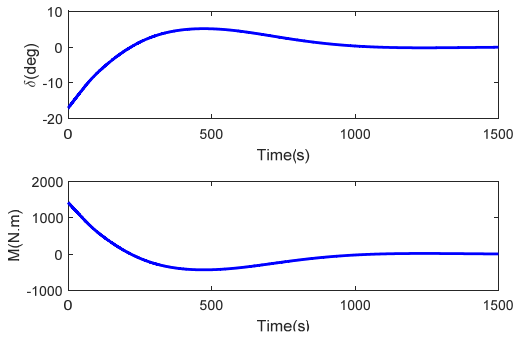
شکل ۱۴- تغییرات ورودی‌های کنترلی برای کنترلر فازی
