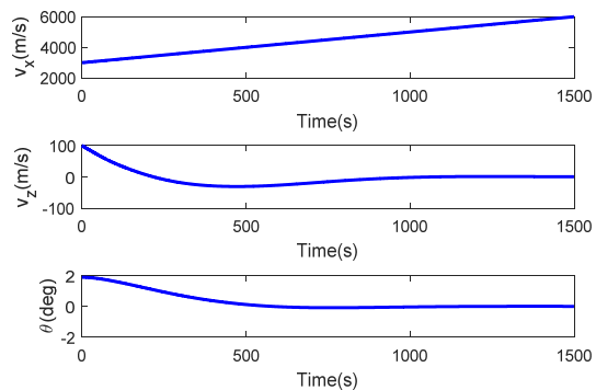
شکل ۱۴- پاسخ زمانی بردارهای وضعیت فضاپیما برای کنترلر فازی
