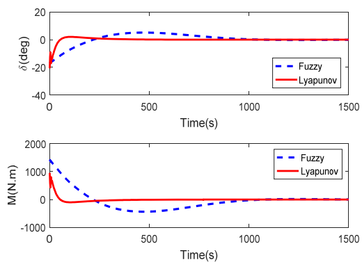
شکل ۲۳- مقایسه تغییرات ورودی‌های کنترلی برای کنترلرهای غیرخطی
