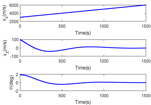
شکل ۵- پاسخ زمانی بردارهای وضعیت فضاپیما برای کنترلر کلاسیک
