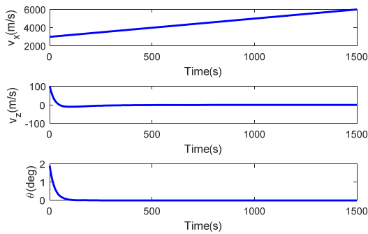
شکل ۱۶- پاسخ زمانی بردارهای وضعیت فضاپیما برای کنترلر لیاپانوف
