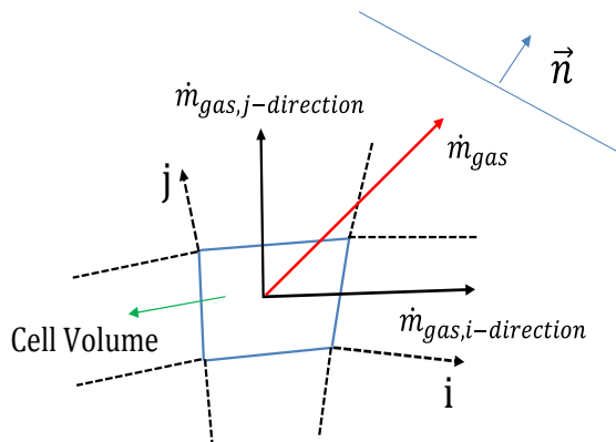
شکل ۹- تجزیه بردار جهت گاز پیرولیز به مؤلفه‌های محوری i و j
