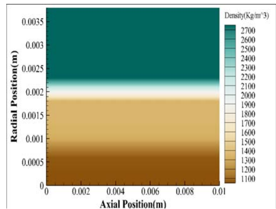
شکل ۲۷- کانتور چگالی عایق کربن فنولیک و بدنه در مدت زمان ۶۰ ثانیه
