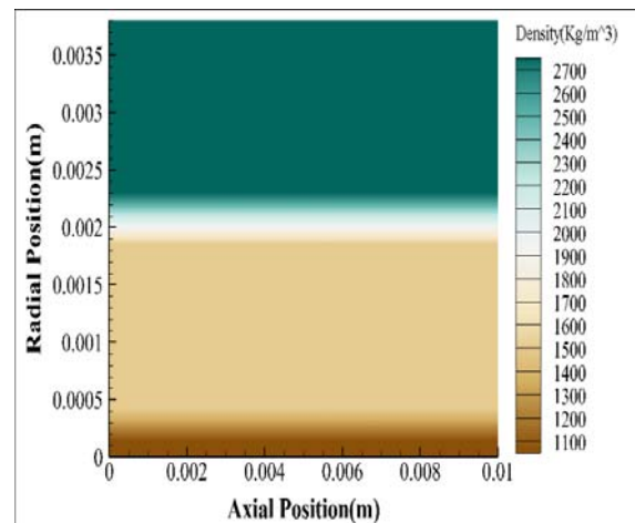
شکل ۲۸- کانتور چگالی عایق ایده‌آل و بدنه در مدت زمان ۶۰ ثانیه
