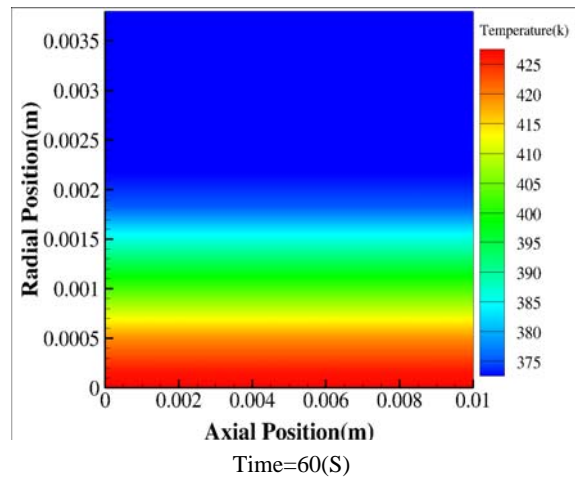
ادامه شکل ۳۰- کانتور دما در مدت زمان ۶۰ ثانیه در عایق ایده‌آل
