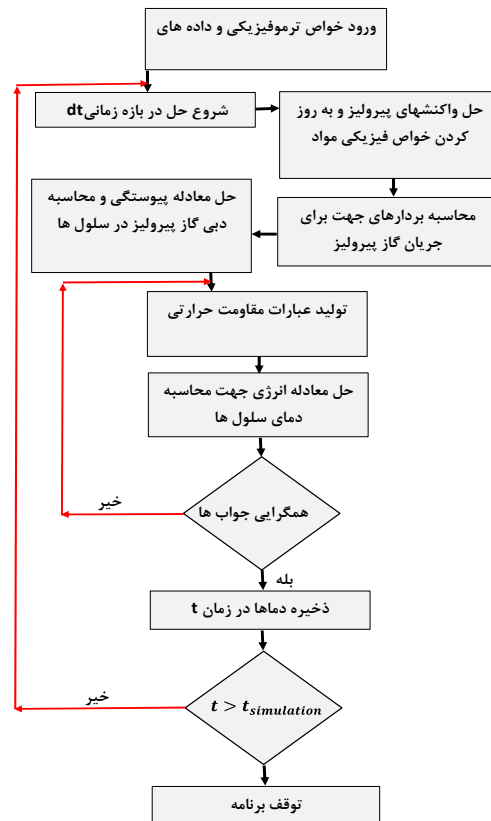
شکل ۱۲- دیاگرام حل معادلات حاکم بر عایق فناشونده
