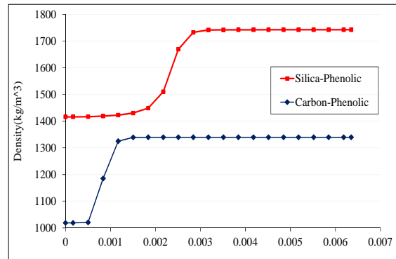
شکل ۲۳- توزیع چگالی در مدت زمان ۵ ثانیه (زمان احتراق) در عایق سلیکا فنولیک و کربن فنولیک در راستای شعاعی
