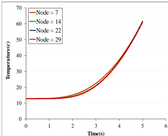
شکل ۱۷- بررسی استقلال حل از شبکه در عایق سلیکافنولیک
