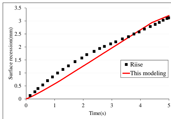
شکل ۱۴- مقایسه نرخ عقب رفت مدل ارائه شده با آزمایش تجربی ریز [۱۳]
