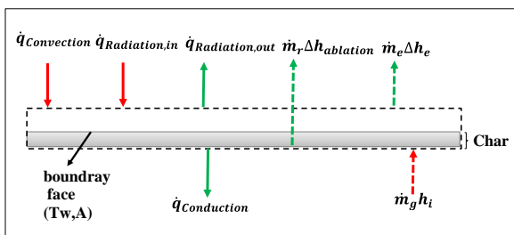
شکل ۱۰- بالانس انرژی و تعادل سطح بر روی سطح ماده فناشونده
