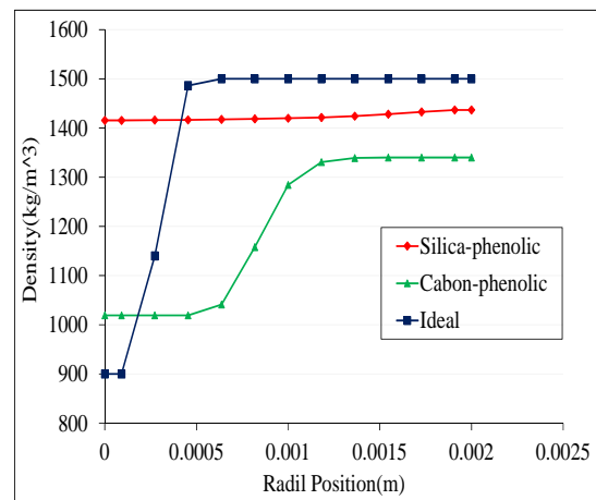
شکل ۲۹- توزیع چگالی در راستای شعاعی در سه دعایق بعد از ۶۰ ثانیه
