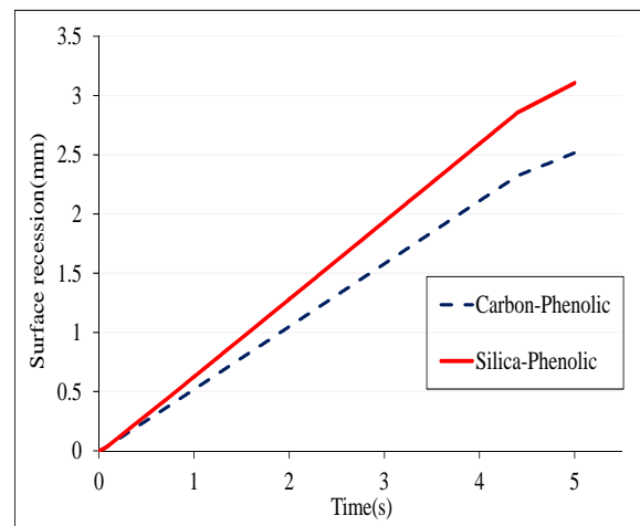
شکل ۲۰- مقایسه میزان پسروی دو عایق کربن فنولیک و سلیکافنولیک
