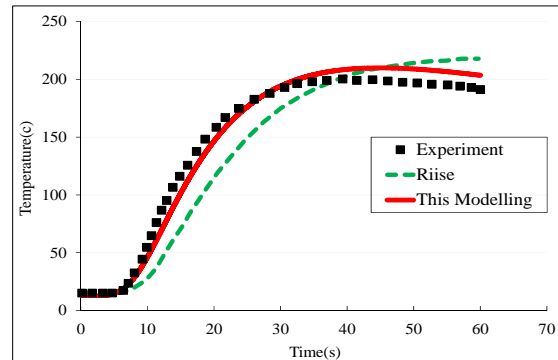
شکل ۱۳- تاریخچه دمای پشت در عایق سلیکا-فنولیک و مقایسه با نتایج تجربی و مدل سازی ریز [۱۳]
