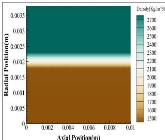
شکل ۲۶- کانتور چگالی در عایق سلیکافنولیک و بدنه در مدت زمان ۶۰ ثانیه
