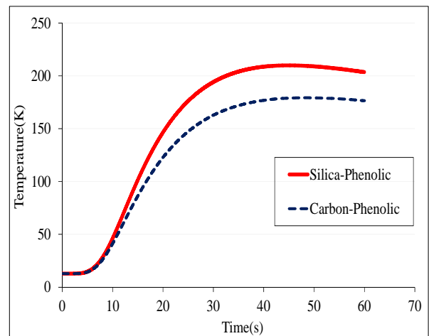
شکل ۱۹- مقایسه تاریخچه دمای پشت در عایق سلیکا-فنولیک و کربن فنولیک
