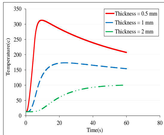
شکل ۳۱- مقایسه تاریخچه دمای پشت در عایق ایده‌آل، در ضخامت‌های ۰.۵، ۱ و ۲ میلی‌متر
