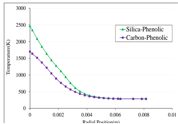
شکل ۲۴- توزیع دما در مدت زمان ۵ ثانیه (زمان احتراق) در عایق سلیکا فنولیک و کربن فنولیک در راستای شعاعی
