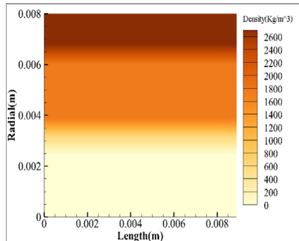
شکل ۱۵- توزیع چگالی در عایق سلیکا فنولیک با پیرولیز و پسروی در مدت زمان احتراق (۵ ثانیه)
