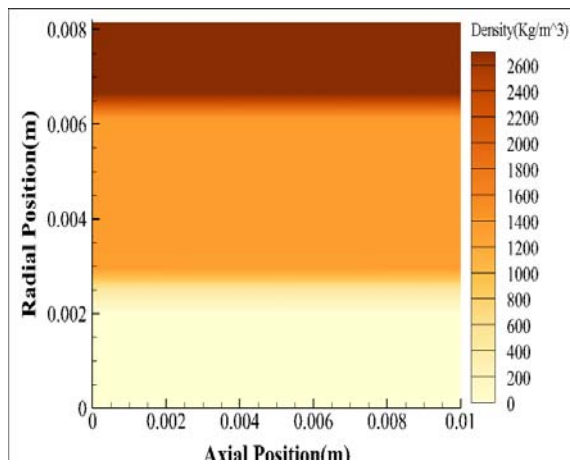
شکل ۲۱- توزیع چگالی در مدت زمان احتراق ۵ ثانیه در عایق کربن فنولیک با در نظر گرفتن پسروی عایق
