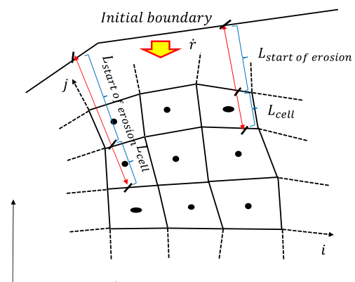
شکل ۱۱- طول مورد استفاده جهت محاسبه پسروی در سلول
