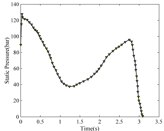
شکل ۳۳- نمودار فشار-زمان تست تجربی انجام شده
