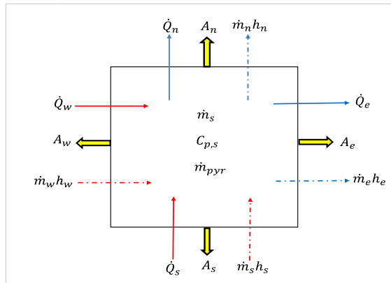
شکل ۸- پایستگی انرژی برای یک حجم کنترل داخلی [۶]
