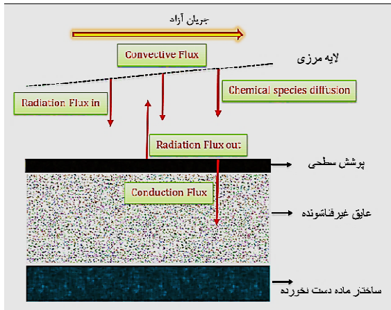
شکل ۷- شماتیک عملکرد سپرهای حرارتی غیرفناشونده [۱۰]
