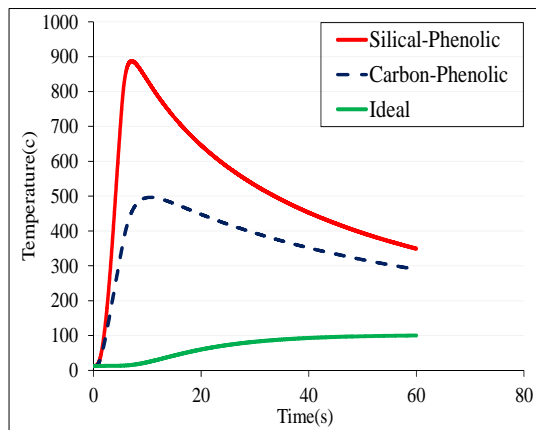
شکل ۲۵- مقایسه تاریخچه دمای پشت در سه عایق سلیکا-فنولیک، کربن فنولیک و عایق ایده آل در ضخامت ۲ میلی‌متر
