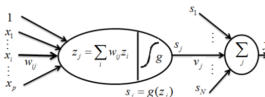
شکل ۶ - ساختار کلی نرون
