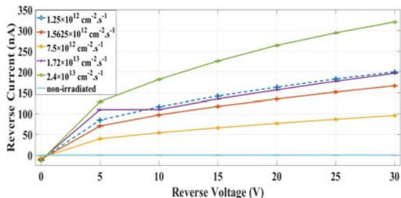
شکل ۱۵- تغییرات جریان نشتی فوتودیودهای نوع BPW34 پس از تابش با شارهای تابشی مختلف از پروتون‌های 30 \text{ MeV}
