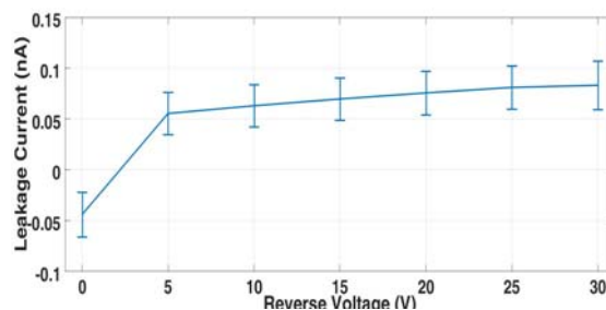
شکل ۱۲- منحنی متوسط جریان نشتی بر حسب ولتاژ فوتودیودهای BPW34 در شدت نوری صفر
