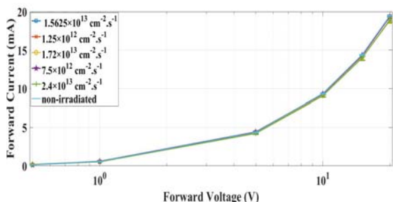
شکل ۱۶- جریان مستقیم فوتودیودهای نوع BPW34 پس از تابش با شارهای تابشی مختلف از پروتون‌های 30 \text{ MeV}
