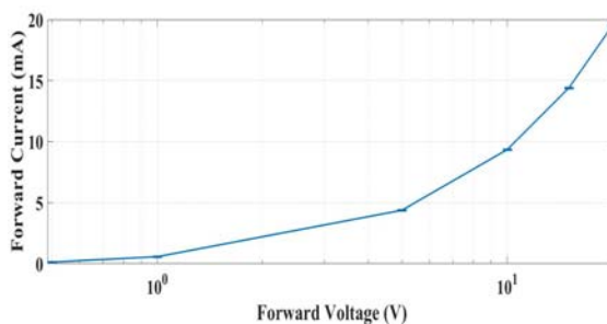
شکل ۱۳- منحنی I-V میانگین قبل تابش برای فوتودیودهای BPW34
