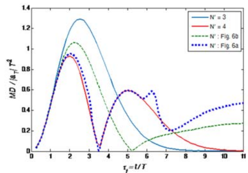
شکل ۲۰ - فاصله خطای بی‌بعد ناشی از مانور هدف با ضریب ناوربری متغیر فرم ب شکل ۶ ( \xi^* = 3^\circ )
