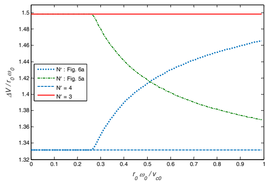
شکل ۳۴- نمایش بی‌بعد انتگرال قدر مطلق دستور شتاب برحسب r_0 \omega_0 / v_{c0} ناشی از انحراف سمت اولیه با فرض سیستم کنترل ایده‌آل به ازای ضریب ناوبری ثابت و متغیر ( \xi^* = 15^\circ )
