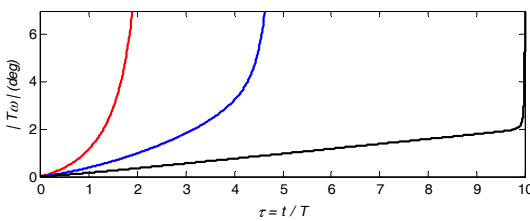
شکل ۳- رفتار زاویه بردار سرعت نسبت به خطدید و نرخ چرخش خطدید بی‌بعد در حالت هدف با مانور ثابت تحت قانون هدایت تناسبی حقیقی ( n = 5, N' = 3, \hat{a}_T = 1, \hat{v}_{c0} = 41.4 )
