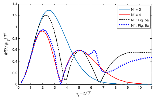
شکل ۱۹ - فاصله خطای بی‌بعد ناشی از مانور هدف با ضریب ناوربری متغیر فرم الف شکل ۶ ( \xi^* = 3^\circ )
