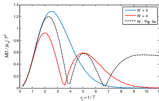
شکل ۱۶ - فاصله خطای ناشی از مانور هدف ثابت با ضریب ناوربری متغیر فرم الف شکل ۵ ( \xi^* = 3^\circ )
