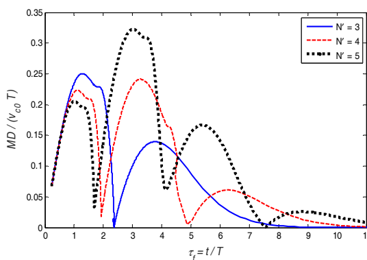
شکل ۴- فاصله خطای بی‌بعد ناشی از انحراف سمت اولیه در مختصات قطبی ( n = 5, \hat{v}_{c0} = 1 )
