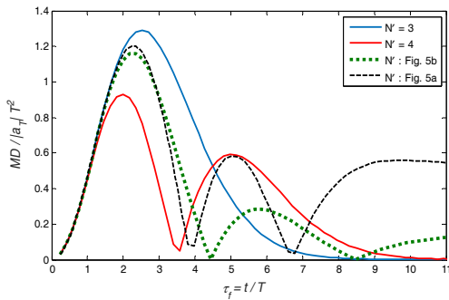
شکل ۱۷ - فاصله خطای ناشی از مانور هدف ثابت با ضریب ناوربری متغیر فرم ب شکل ۵ ( \xi^* = 7.5^\circ )
