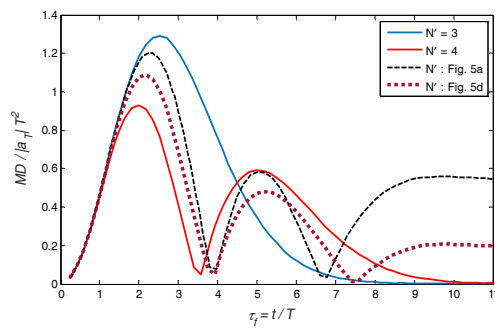
شکل ۱۸ - فاصله خطای ناشی از مانور هدف ثابت با ضریب ناوربری متغیر فرم د شکل ۵ ( \xi^* = 4^\circ )
