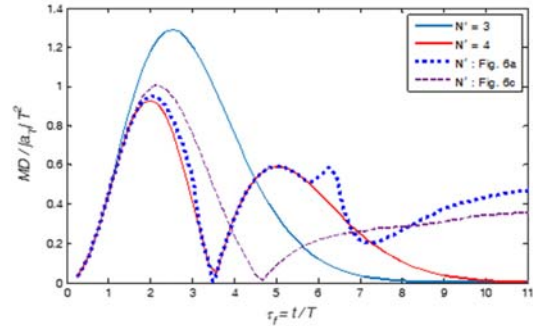
شکل ۲۱- فاصله خطای بی‌بعد ناشی از مانور هدف با ضریب ناوبری متغیر فرم ج شکل ۶ ( \xi^*_{min} = 1^\circ, \xi^*_{max} = 4^\circ )
