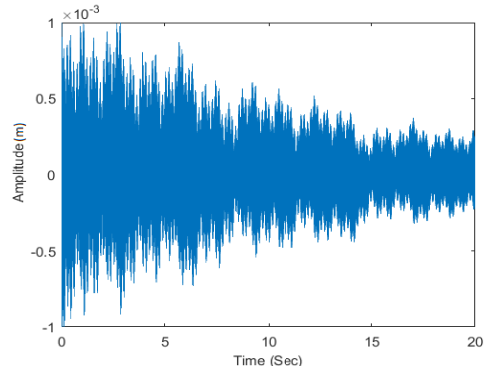
شکل ۲- جابه‌جایی سازه یک سر گیردار ساندویچی بدون اثر وصله‌های پیزوالکتریک
