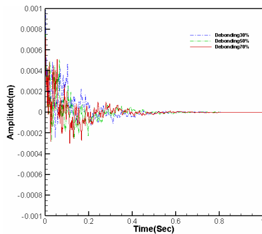
شکل ۹- اثرات ناپیوستگی بر جابه‌جایی سازه یک سر گیردار ساندویچی با اثر وصله پیزوالکتریک
