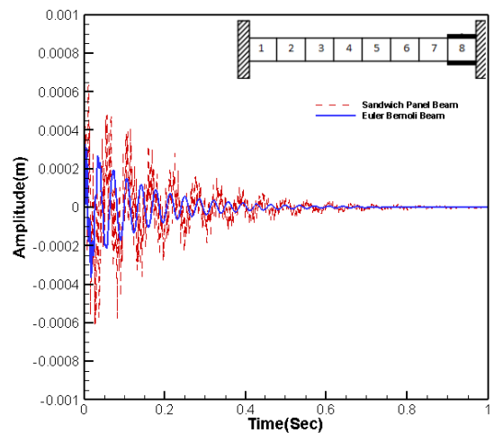
شکل ۲۰- جابه‌جایی سازه دو سر گیردار با اثر وصله پیزوالکتریک بر روی المان انتهایی
