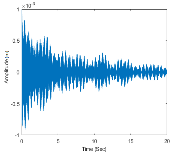
شکل ۱۹- جابه‌جایی سازه دو سر گیردار ساندویچی بدون اثر وصله‌های پیزوالکتریک
