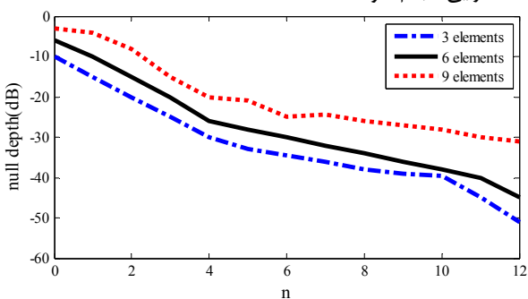
شکل ۵- نمودار مقایسه‌ای عمق صفر الگوی تشعشعی بر حسب مقدار سمت‌گرایی به ازای تعداد عنصرهای مختلف
