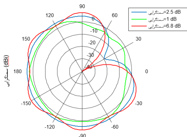
شکل ۳- مقدار عمق صفر الگوی تشعشعی به ازای مقادیر مختلف سمت‌گرایی وقتی تغذیه‌ی یکی از عنصرها خاموش باشد.
