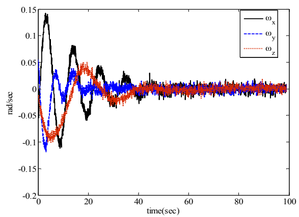
شکل ۱۳- تغییرات سرعت زاویه‌ای پلتفرم با کنترل‌کننده PD در شرایط تعادل پایدار
