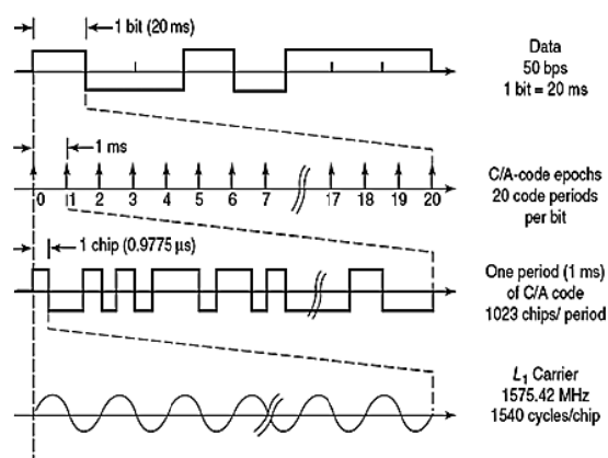
شکل ۴- مراحل تولید سیگنال ارسالی ماهواره
