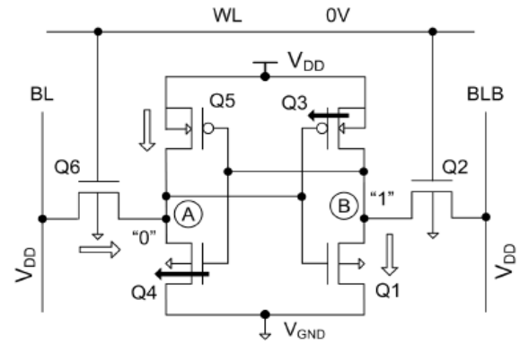
شکل ۱- مدار داخلی یک سلول حافظه SRAM
