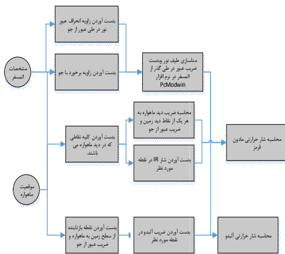
شکل ۱۲- فلوجارت نحوه محاسبه شار حرارتی مادون قرمز و آلبدو
