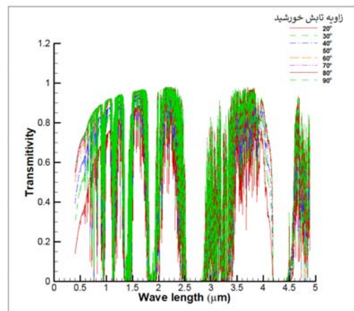
شکل ۵- تغییرات ضریب عبور نور از اتمسفر بر حسب طول موج برای زوایای تابشی مختلف به زمین
