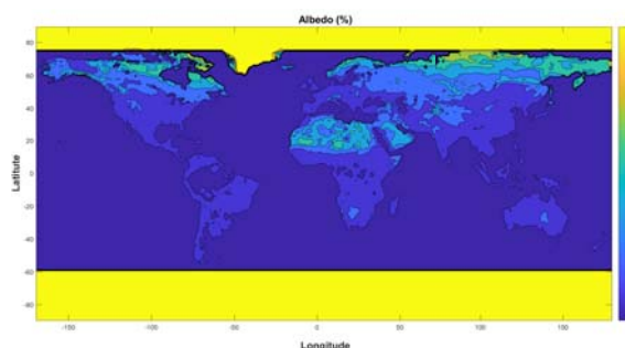
شکل ۷- کانتور توزیع ضریب آلبدو در نقاط مختلف سطح کره زمین
