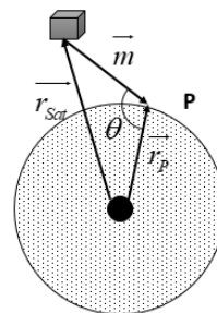
شکل ۱- بردار موقعیت نقطه P و مکان ماهواره
