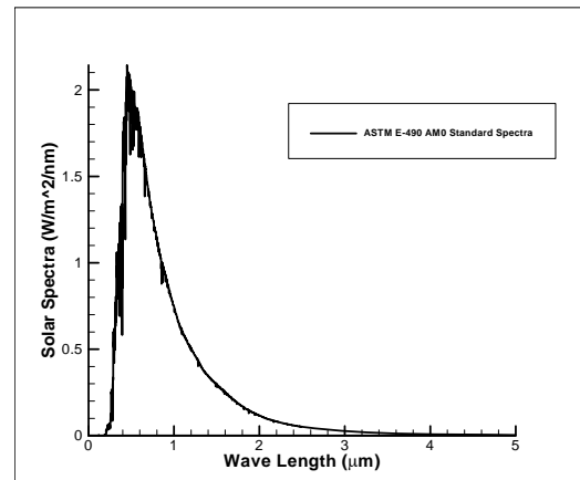
شکل ۴- توزیع رادیانس خورشیدی بر حسب طول موج مطابق استاندارد ASTM-E490
