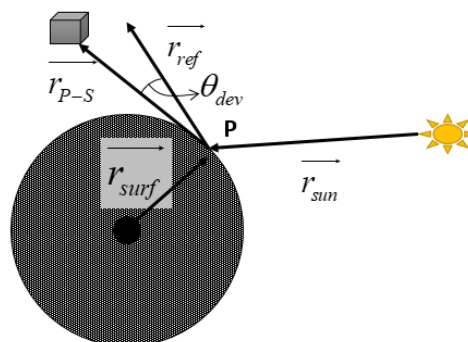
شکل ۸- بردارهای تابش و بازتابش نور خورشید
