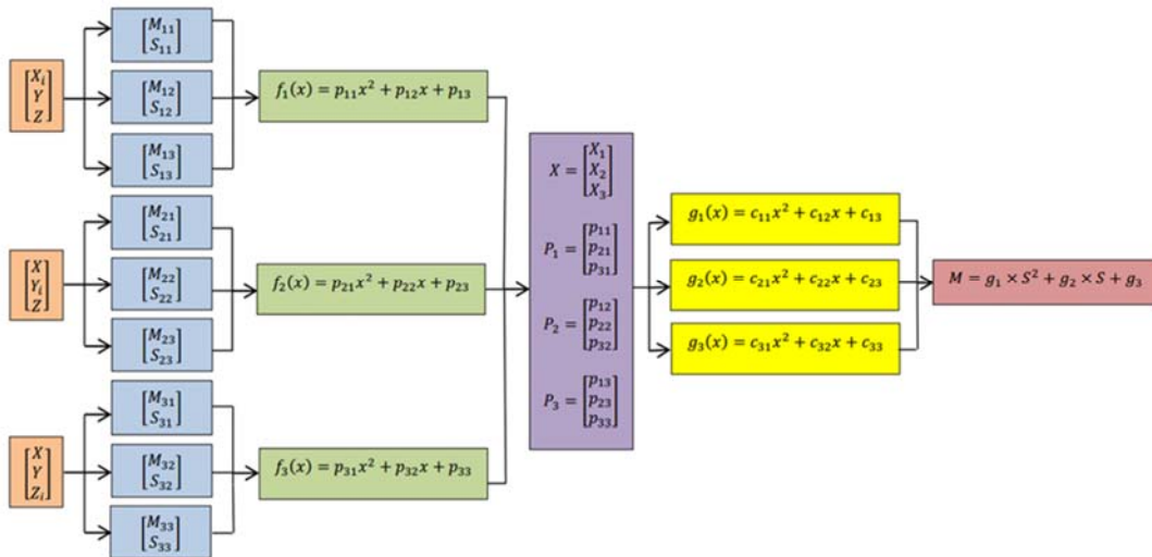
شکل ۲- روش وابستگی تو در تو به صورت بلوک دیاگرام
