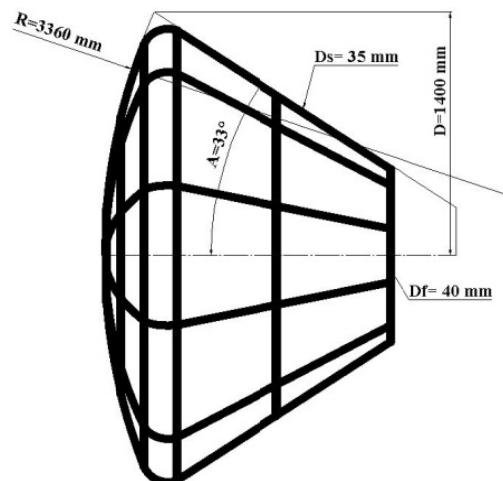
شکل ۴- سازه داخلی کپسول فضایی
