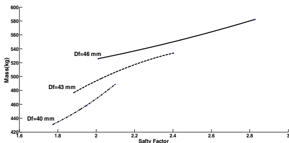
شکل ۹- برازش منحنی بر روی نقاط در سه حالت مختلف قطر فریم
