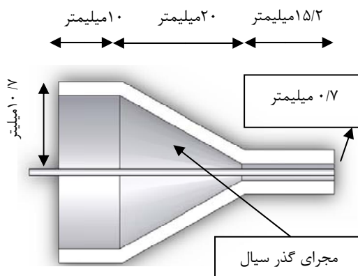
شکل ۳- هندسه نازل
