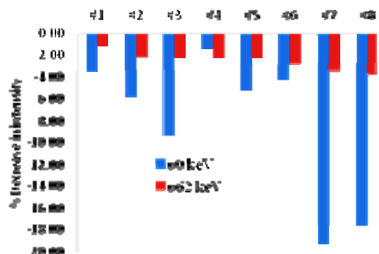
شکل ۶- مقایسه میزان افت ایجاد شده ناشی از حفاظت ساندویچ پل‌های سازهای در برابر تابش دو سطح انرژی ۶۰ keV و ۶۶۲ keV
