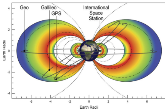
شکل ۱- موقعیت کمربندهای داخلی و خارجی و آن و مدارهای ماهواره‌ای [۵]
