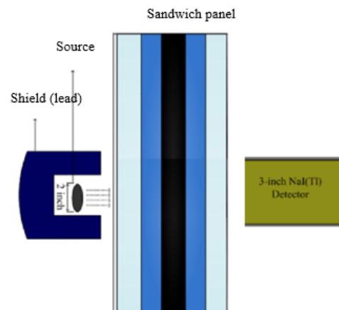
شکل ۵- چیدمان آزمون برای اندازه‌گیری میزان حفاظت
