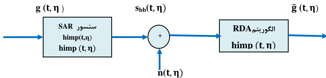
شکل ۹- مدل پیشنهادی سامانه تصویربرداری g(t, \eta)
