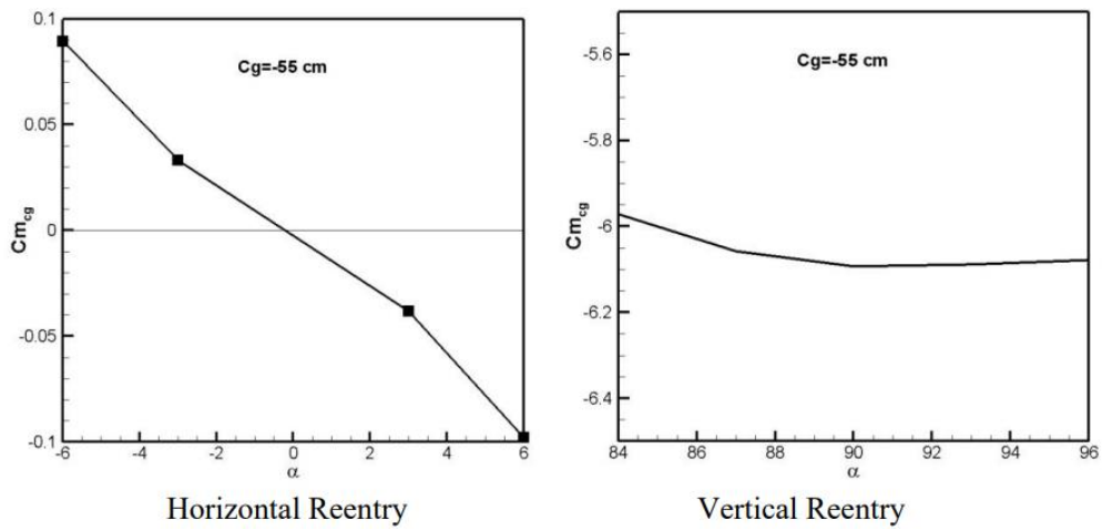
شکل ۴- توزیع مقدار ضریب گشتاور پیچشی برای بازایی افقی و عمودی برای x_{cg} = -0.55m
