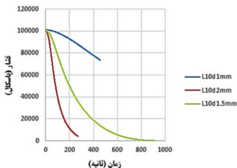
شکل ۱۴ - تغییرات فشار در دو نقطه میانی نمونه‌برداری با طول المان ۱۰ میلی‌متر و قطر سوراخ ۱، ۱/۵ و ۲ میلی‌متر
