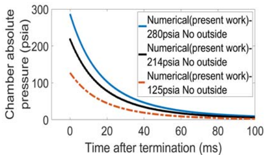
شکل ۹. نمودار تغییرات فشار برحسب زمان برای فشارهای اولیه ۲۸۰، ۲۱۴ و ۱۲۵
