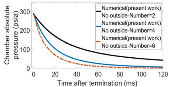
شکل ۱۹. نمودار تغییرات فشار برحسب زمان برای تعداد دریچه‌های ۲، ۴ و ۶
