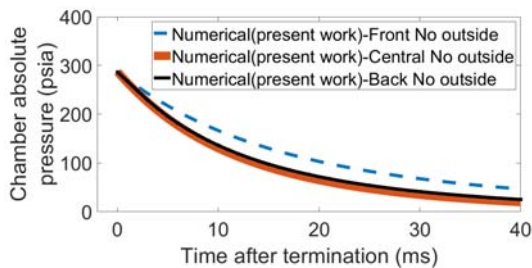
شکل ۲۰. نمودار تغییرات فشار برحسب زمان برای محل قرارگیری دریچه‌ها در جلو، وسط و عقب موشک
