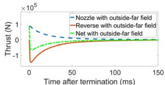
شکل ۶. نمودار تغییرات تراست برحسب زمان برای فشار اولیه ۲۸۰ psi برای حالت Pressure_farfield و با محیط بیرون
