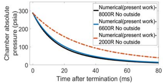
شکل ۱۷. نمودار تغییرات فشار برحسب زمان برای دماهای اولیه ۲۰۰۰، ۶۶۰۰ و ۸۰۰۰ رانکین
