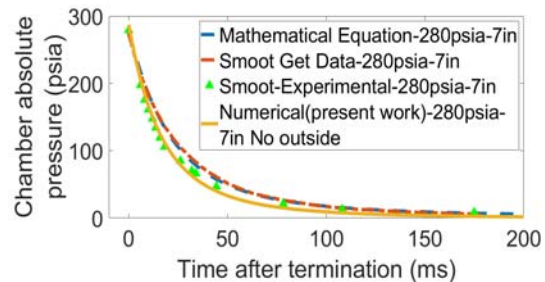
شکل ۷. نمودار تغییرات فشار برحسب زمان برای فشار اولیه ۲۸۰ psi بدون محیط بیرون
