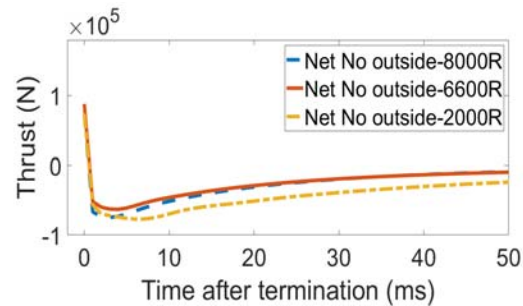
شکل ۱۸. نمودار تغییرات تراست کل برحسب زمان برای دماهای اولیه ۲۰۰۰، ۶۶۰۰ و ۸۰۰۰ رانکین
