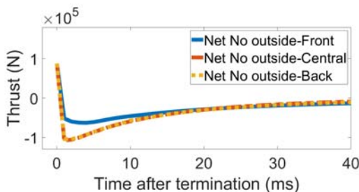
شکل ۲۱. نمودار تغییرات تراست کل برحسب زمان برای محل قرارگیری دریچه‌ها در جلو، وسط و عقب موشک
