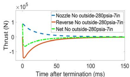
شکل ۸. نمودار تغییرات تراست برحسب زمان برای فشار اولیه ۲۸۰ psi بدون محیط بیرون
