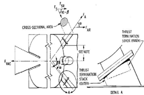
شکل ۱. شکل شماتیکی از موتور سوخت جامد بعد از باز شدن درپچه‌های تراست معکوس و دودکش‌های داخلی و خارجی [۱۱]
