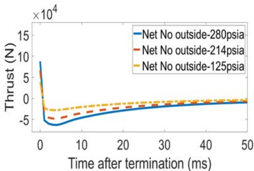
شکل ۱۰. نمودار تغییرات تراست کل برحسب زمان برای فشارهای اولیه ۲۸۰، ۲۱۴ و ۱۲۵
