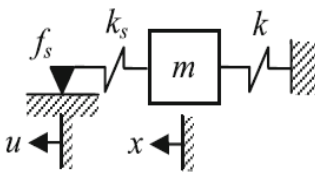
شکل ۲- المان جنکینز در یک سیستم یک درجه آزادی
