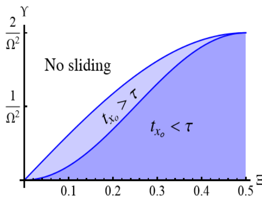
شکل ۴- نواحی وقوع یا عدم وقوع لغزش
