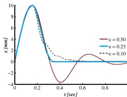
شکل ۱۱- پاسخ زمانی جابه‌جایی به شرط اولیه سرعت در نسبت سختی‌های مختلف
