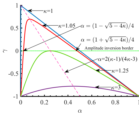
شکل ۳- منحنی مشخصه پاسخ ضربه المان جنکینز
