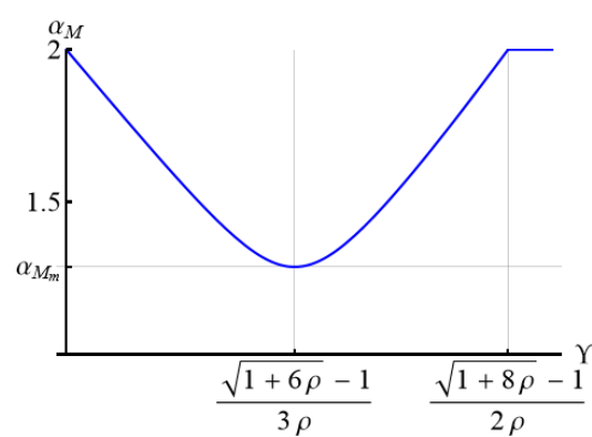
شکل ۸- تغییرات بیشینه طیف پاسخ شوک بر حسب آستانه اصطکاک با فرض وابستگی خطی نسبت سختی و آستانه اصطکاک
