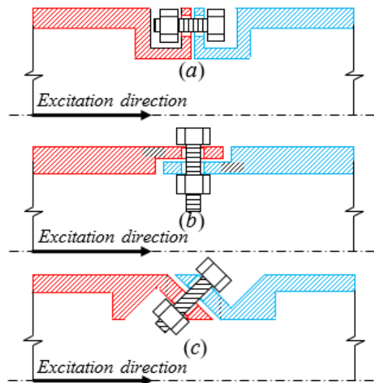
شکل ۱- هندسه‌های گوناگون اتصال پیچ، (a) اتصال عمود، (b) اتصال موازی و (c) اتصال اُریب
