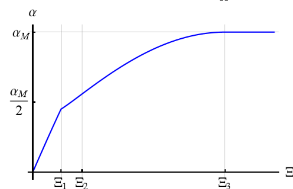
شکل ۵- طیف پاسخ شوک
