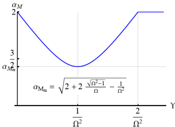
شکل ۶- تغییرات بیشینه طیف پاسخ شوک بر حسب آستانه اصطکاک با فرض عدم وابستگی نسبت سختی و آستانه اصطکاک
