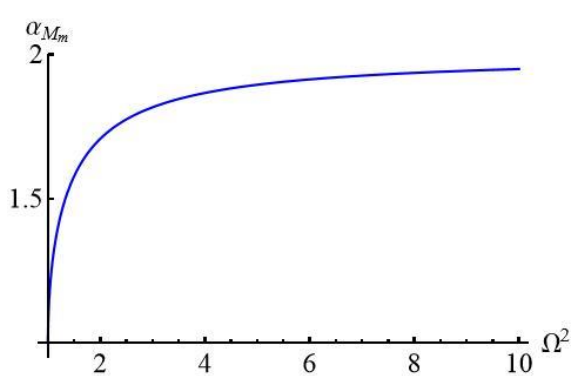
شکل ۷- تغییرات کمینه‌ی بیشینه طیف پاسخ شوک بر حسب نسبت سختی
