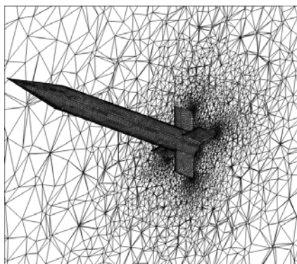
شکل ۲- شبکه تولید شده حول مدل سه‌بعدی استاندارد پیسیک فیبر
