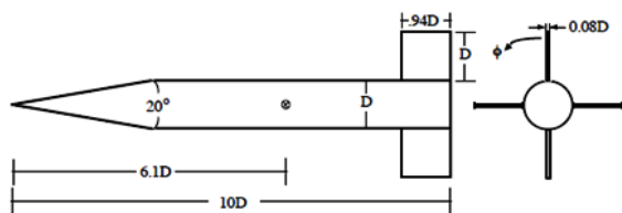
شکل ۱- هندسه سه‌بعدی مدل استاندارد پیسیک فیبر
