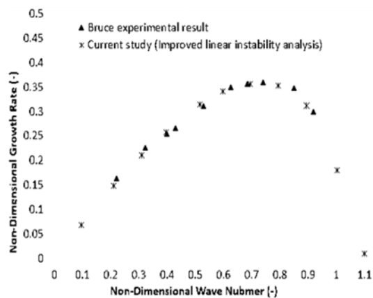
شکل ۹- مقایسه متحنی نرخ رشد بی‌بعد بر حسب عدد موج حاصل از روش
