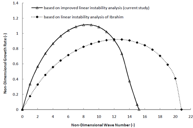
شکل ۷ - مقایسه منحنی نرخ رشد موج به روش بهبودیافته خطی با روش خطی مرسوم برای آنزکتور طراحی شده آزمایشگاهی در شرایط We_{ix} = 3390 ، We_{ox} = 1.03 ، We_{is} = 347 ، We_{os} = 0 ، g_i = g_o = 0.00122 ، h = 0.78 ، n = 0
