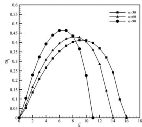
شکل ۱۰- تأثیر زاویه پاشش روی توزیع نرخ رشد موج بی‌بعد در شرایط
