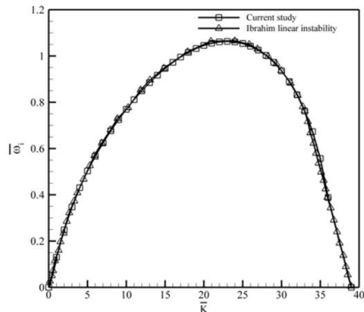
شکل ۸- مقایسه متحنی نرخ رشد موج به روش بهبودیافته با روش خطی مرسوم
