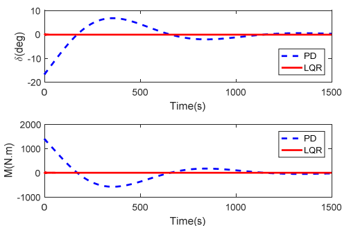
شکل ۱۳- مقایسه تغییرات ورودی‌های کنترلی برای کنترلرهای خطی
