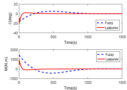
شکل ۲۵- مقایسه تغییرات ورودی‌های کنترلی برای کنترلرهای غیرخطی
