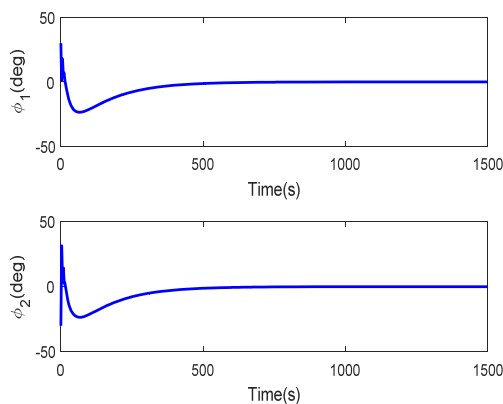
شکل ۲۴- پاسخ زمانی وضعیت پاندولها در مرجع [۱۶]
