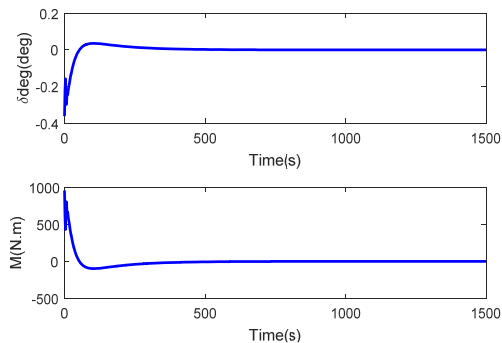
شکل ۱۹- تغییرات ورودی‌های کنترلی برای کنترل لیاپانوف
