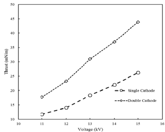
شکل ۱۲- مقایسه نمودار تراست-ولتاژ برای دو پیکربندی
