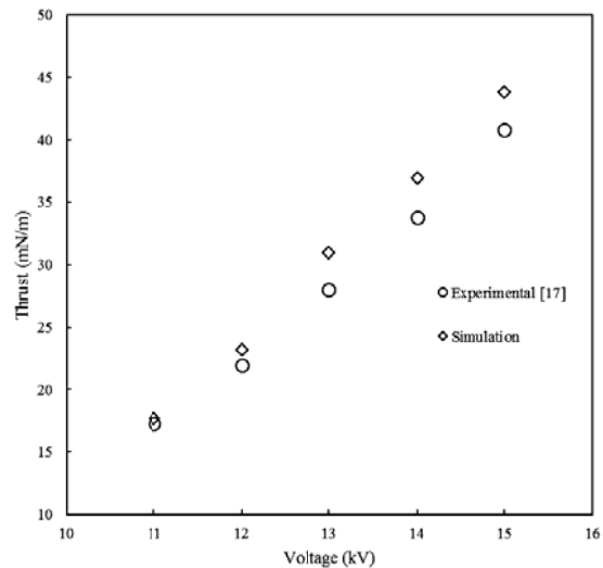
شکل ۶- نمودار نیروی پیشران بر حسب ولتاژ در پیکربندی دو کاتده
