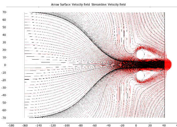
شکل ۸- خطوط جریان در ولتاژ 12 \text{ kV}
