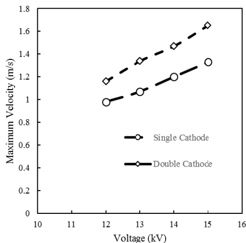
شکل ۱۰- نمودار بیشینه سرعت بر حسب ولتاژ
