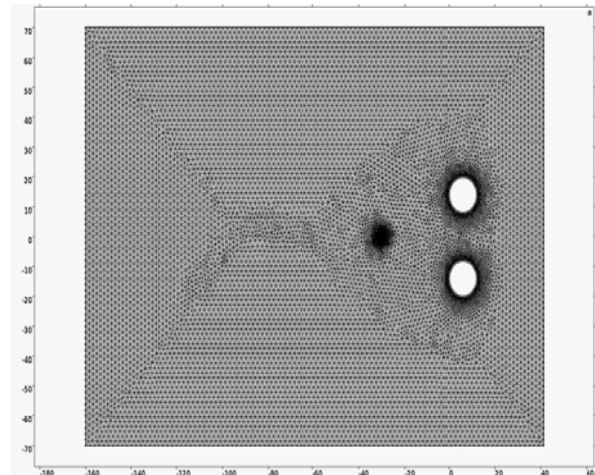
شکل ۳- شبکه بندی مسئله
