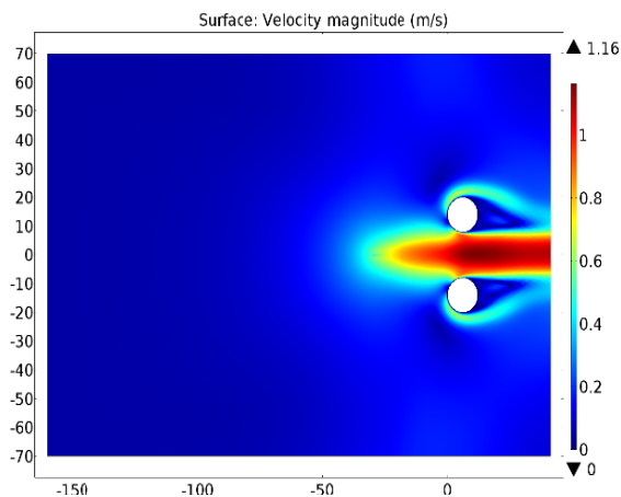
شکل ۷- کانتور سرعت در ولتاژ 12 \text{ kV}
